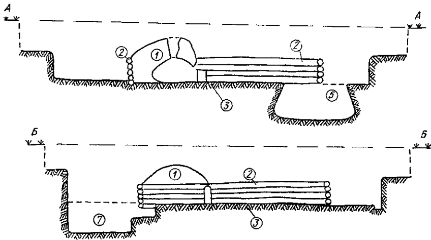
Рис. 5. С. Волицеве. План і профіль житла № 13:
