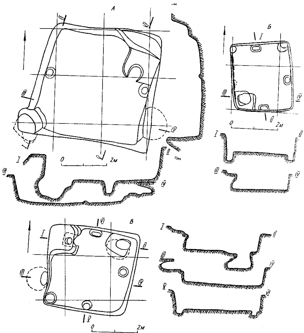
Рис. 3. Городище Новотроїцьке (волинцівський етап). Житла різної конструкції: А — ґрунтова; Б — каркасна; В — зрубна.
