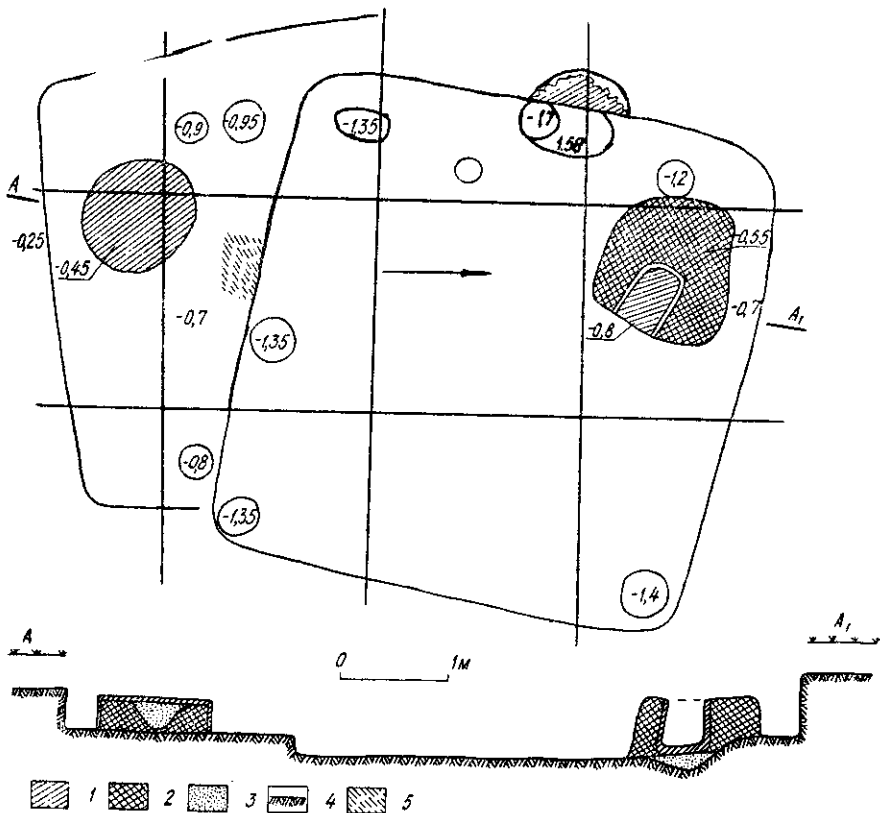
Рис. 4. Волинцеве. План і профіль житла № 39:
