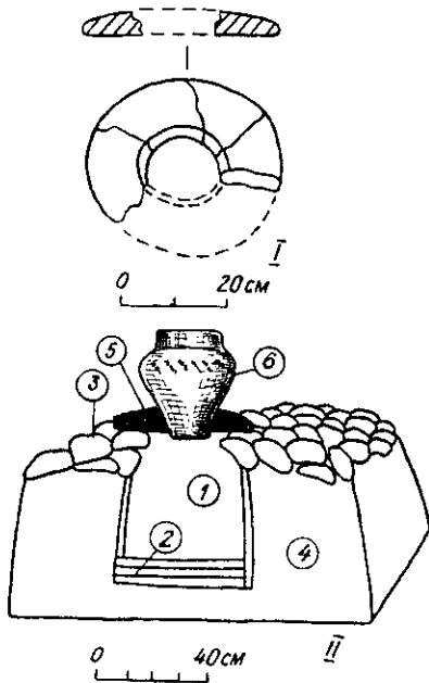
Рис. 8. Волинцеве. I — глиняна деталь верхньої частини печі житла № 39; II — реконструкція печі житла № 39:
