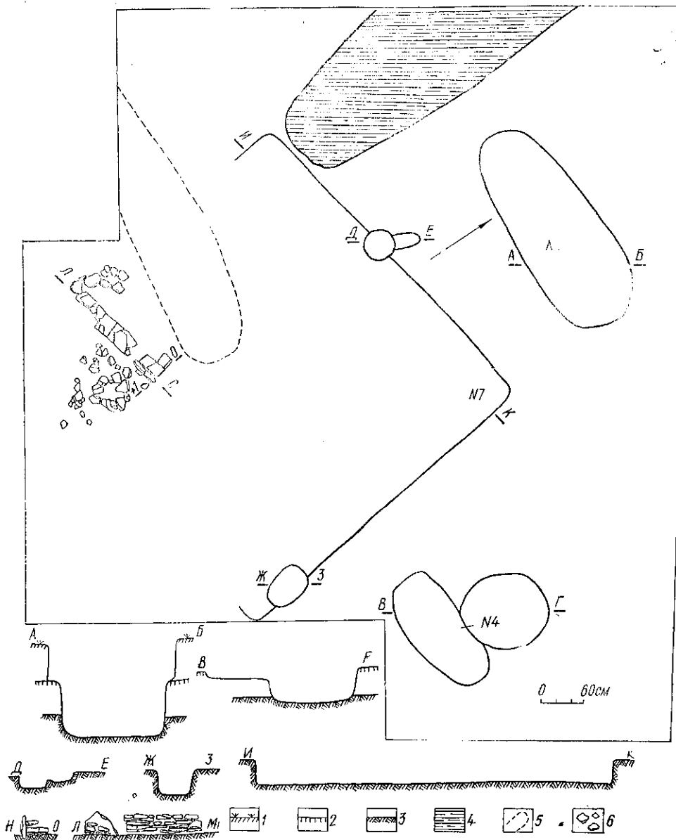
Рис. 5. План розкопа і профілі об'єктів західної ділянки городища:
