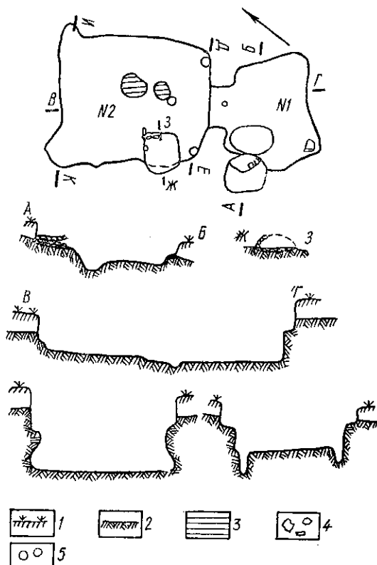
Рис. 6. План та розрізи жител № 1 і № 2:
