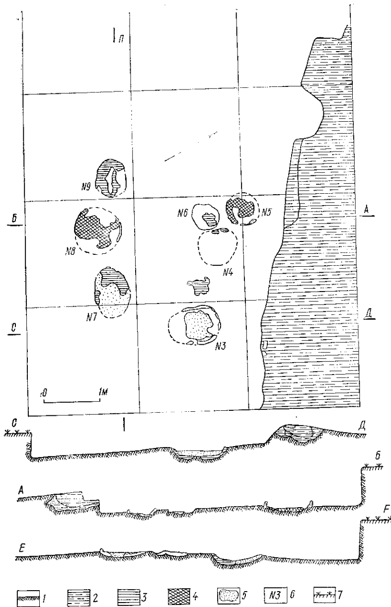
Рис. 8. Плани та розрізи печей у східній частині городища:
