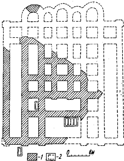
Рис. 5. План фундаментів Кловського собору за розкопками 1974—1975 рр.: 1 — розкопана частина фундаментів храму; 2 — реконструйована частина фундаментів храму.
