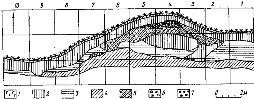
Рис. 7. Розріз західного оборонного валу:
