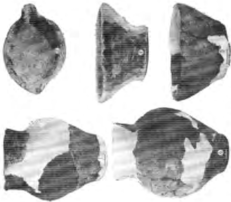
Рис. 13. Ліпна кераміка з комплексу. 1, 4 — горщики; 2 — свігльняк; 3, 5 — чаша
