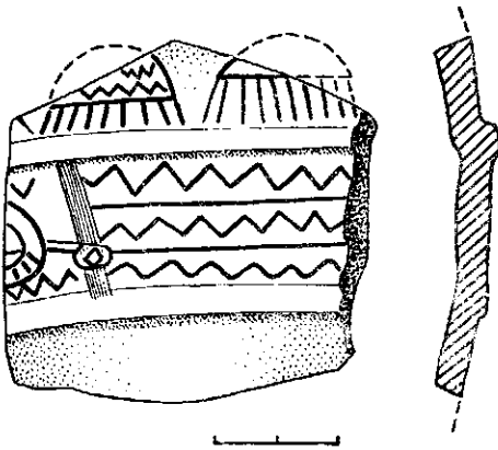
Рис. 10. Фрагмент черняхівської посудини з Тіри.
