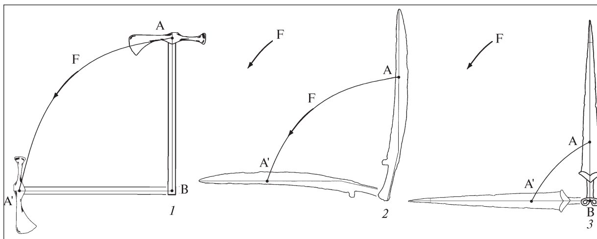
Рис. 4. Реконструкція траєкторії рубального удару різними видами зброї: 1 — сокирою; 2 — односічним мечем; 3 — двосічним мечем ( F — вектор прикладання сили; A-A' — рух центру ваги)
