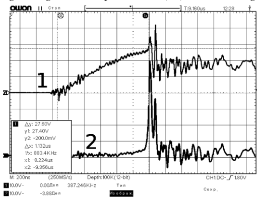
Fig. 4. Oscillograms
