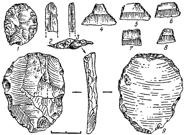
Моспіно. Скребок, ножовидні пластини, трапеції (1—8) мезолітичного часу та скол з черепаховидного нуклеуса (9) муст'єрської епохи.
