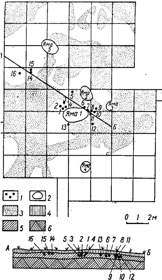
Рис. 2. План і схематичний розріз могильника (по АБ):
