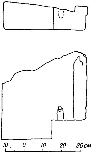
Рис. 8. Фрагмент блока перемички дверного прорізу № 1234. Боковий фасад, план.
