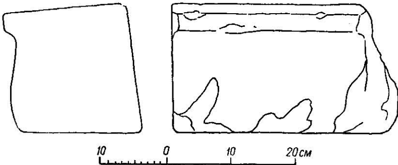
Рис. 12. Вінчаюча частина карниза № 1468 а. Головний фасад, розріз.
