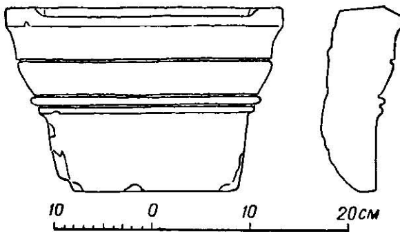
Рис. 5. Капітель пілястра № 1630. Головний фасад, розріз.
