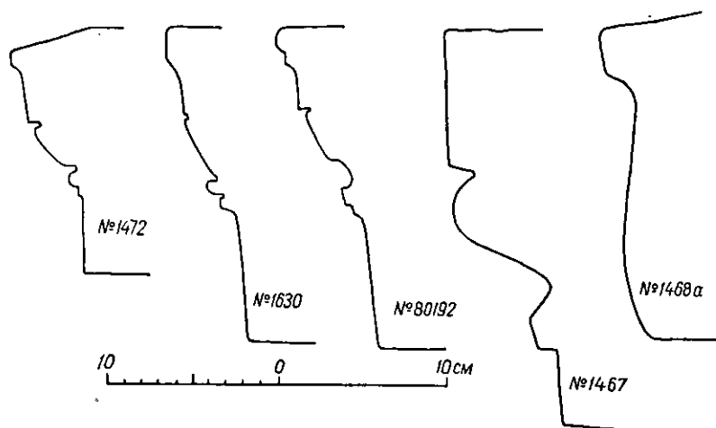
Рис. 13. Обломи капітелей і карниза.
