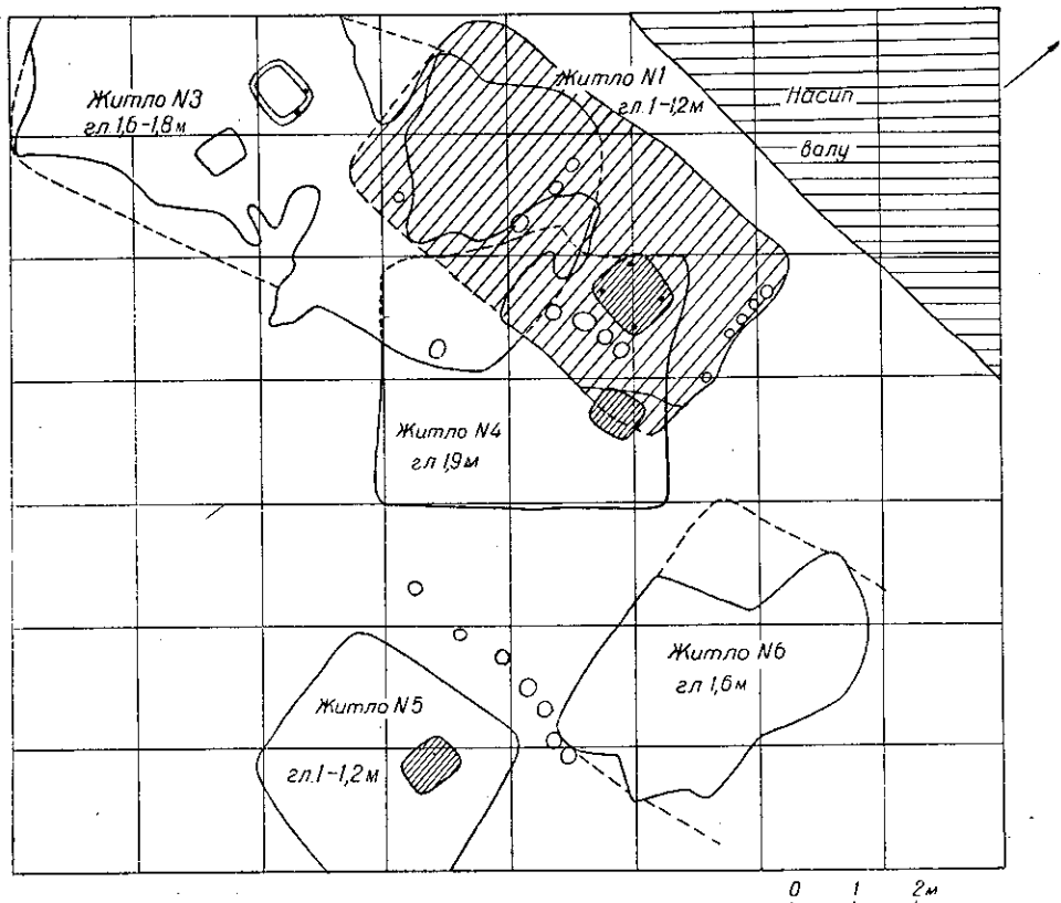
Рис. 3. План та розріз наземних жител на розкопі № 2.
