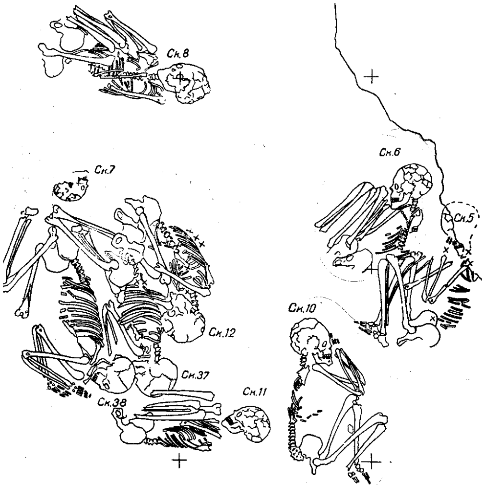
Рис 7. Василівка 3. Поховання 5—8, 10—12, 37, 38. х—кремені вістря і їх уламки.
