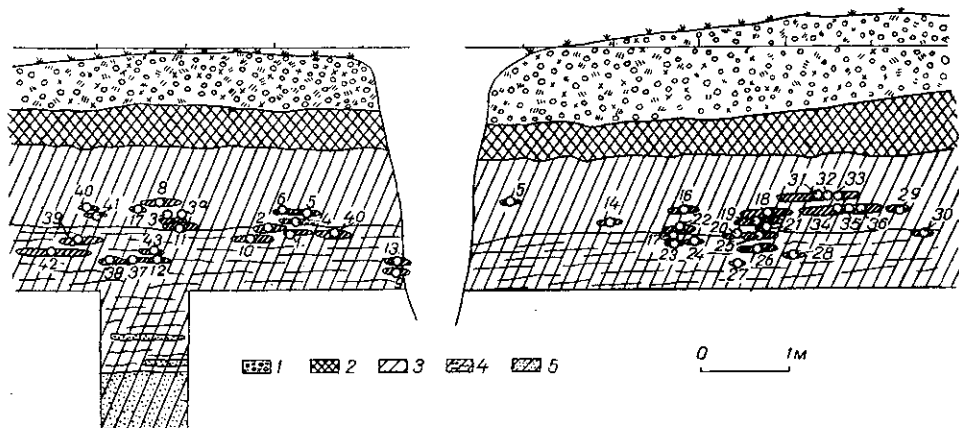
Рис. 1. Василівський третій некрополь; схематичний розріз.
