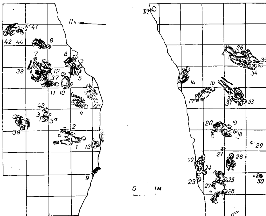
Рис. 2. Василівка 3. Загальний план могильника.
