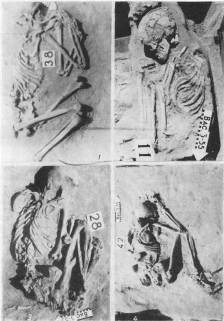
Рис. 3. Василівка 3. Поховання № 38, 11, 28, 42, слабо (1, 4) і сильно (2, 3) скорчені.
