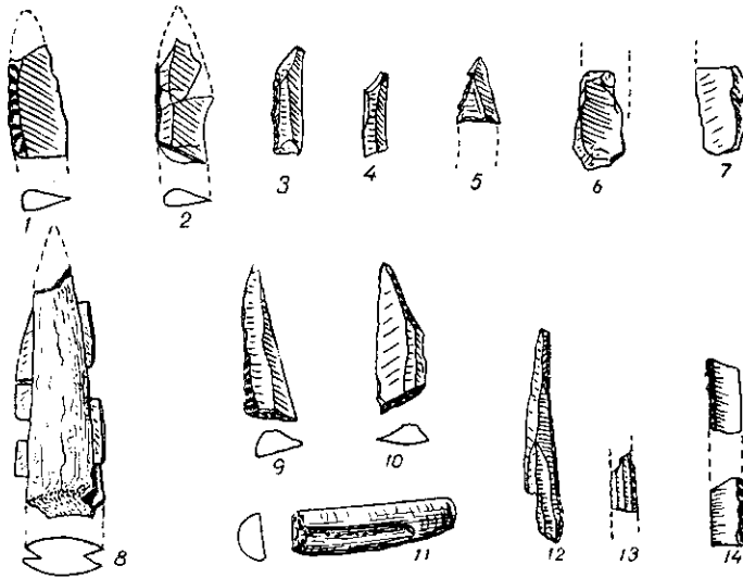
Рис. 5. Крем'яні та кістяні вістря і їх уламки, виявлені при скорчених (1—7) і витягнутих (8—11) похованнях Василівського третього могильника. Вістря з затупленою спинкою Волоського (12) і Василівського першого (13—14) некрополів.
