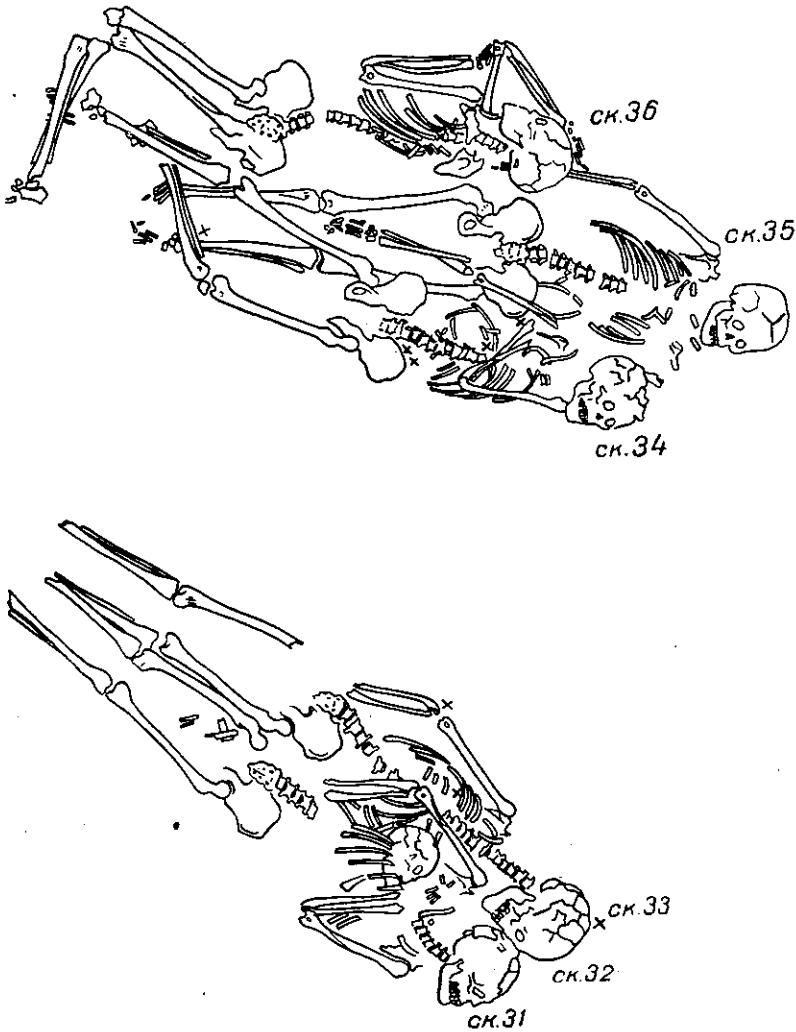
Рис. 10. Василівка 3. Поховання № 31—36. X крем'яні і кістяні знахідки.
