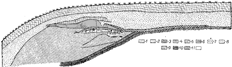
Рис. 3. Розріз розкопу № 1: 1 — шар ґрунтового чорнозему; 2 — культурний шар з великим вмістом золи; 3 — глинобитна підлога житла; 4, 5 — глиняна площадка над насипним шаром; 6 — пропалена глина в основі глинобитної площадки; 7 — залишки кострища; 8 — прошарки сажі в насипу; 9 — насипна земля; 10 — похований чорнозем; 11 — материк.
