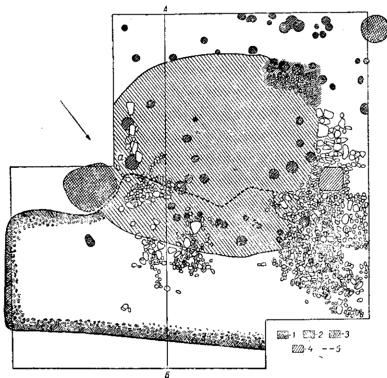
Рис. 2. План розкопу № 1; 1 — глинобитна площадка біля краю городища; 2 — глинобитна підлога житла; 3 — стовпові і господарські ями (літерою „а“ позначена яма, в якій знайдені серпи та рибальський гачок); 4 — вогнищеві спорудження; 5 — край глинобитної площадки, перекритий підлогою житла.
