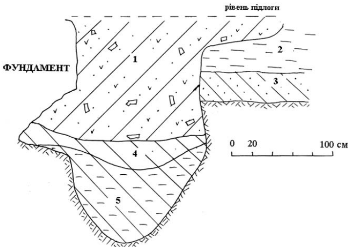
Рис. 14. Новгород-Сіверський. Монументальна споруда. Розріз ями з підбосом: 1 — темно-сірий супісок з цеглою, штукатуркою та горілим деревом; 2 — жовта глина (підсіпка під підлогу); 3 — світло-сірий супісок; 4 — сіро-жовтий супісок; 5 — світло-жовтий плямистий супісок
