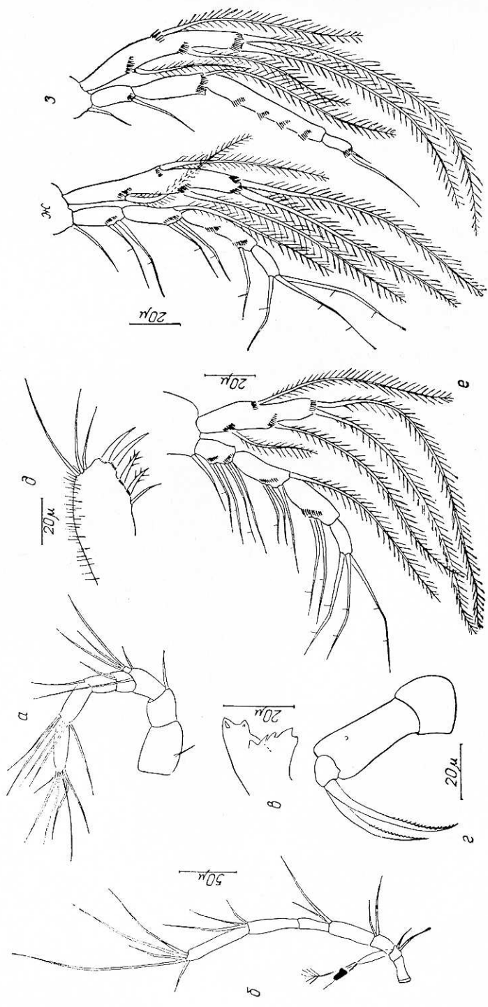
Рис. 2. Vatynella patana ukrainica Monchenko sp. n.
