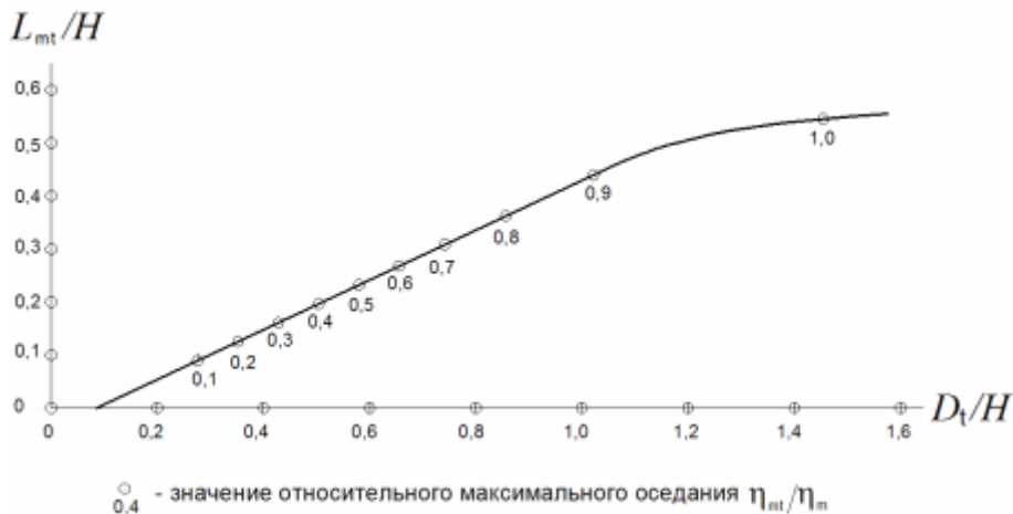
Рис. 5. Общий график относительных максимальных оседаний на стадии формирования мульды
