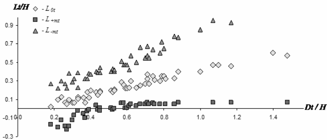
Рис. 3. Распределение L_{mt}/H , L_{-mt}/H , L_{0t}/H от D_t/H для наклонов i_{mt} , i_{-mt} , i_{0t}
