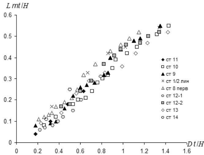
Рис. 2. Распределение L_{mt}/H от D_t/H для оседаний \eta_{mt}
