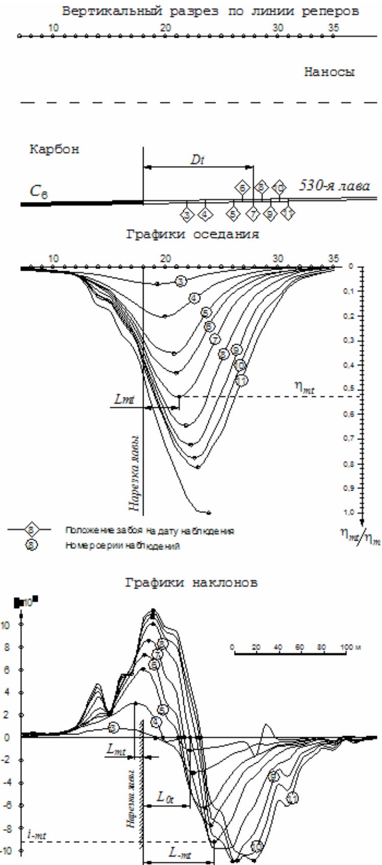
Рис. 1. Графики оседания и наклонов по профильной линии
