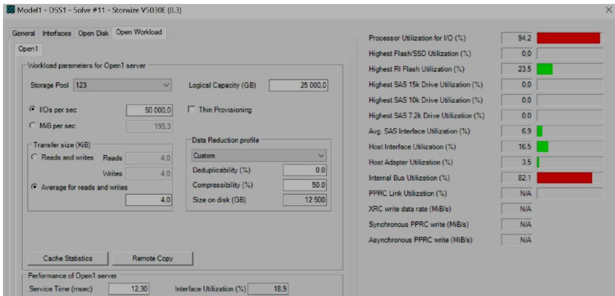
Рис. 15. Вимірювання системи з дисками SSD та програмною компресією
