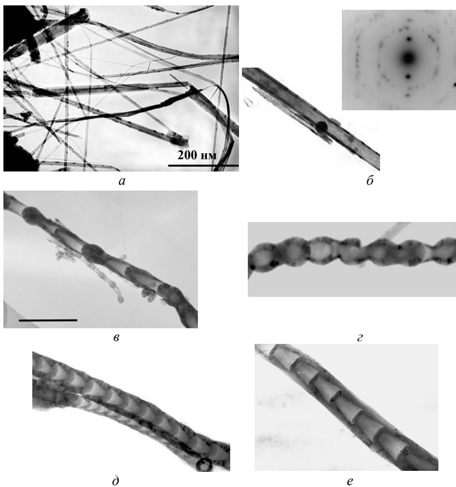
Рис. 5. Типичные формы трубок BN, образующихся из газовой фазы, непрерывного роста ( a — общий вид; б — увеличенный фрагмент и микроэлектронграмма) и прерывистого ( в — е ).
