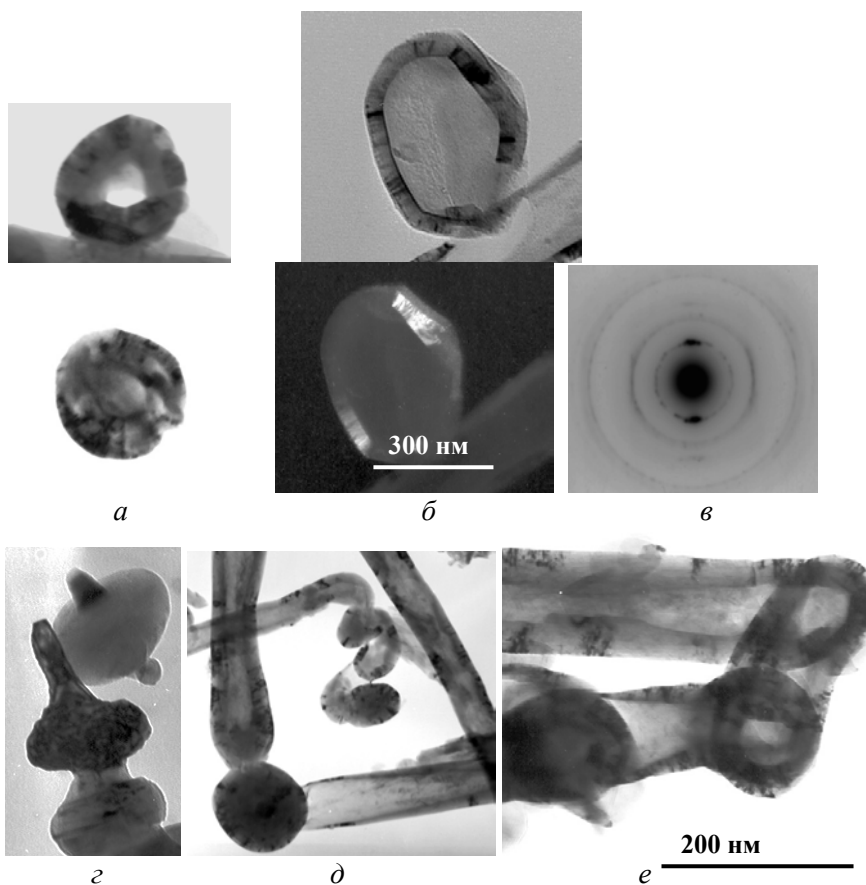
Рис. 2. Типичные морфологические разновидности onionоподобных частиц BN, формирующихся из газовой фазы: a — округлые полые и закрытые; б — ограниченные (типа шапочки) (светло- и темнопольное изображения); в — МЭГ; г — луковичной морфологии; д — в форме шара; е — анизометричные, формирующиеся как элементы коалесценции трубок.
