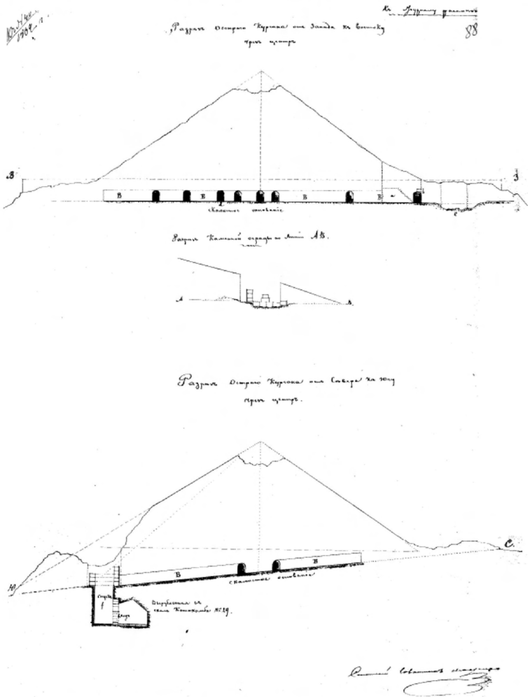
Рис. 3. Острый курган, разрезы [НА ИИМК РАН, ф. 1, 1861 г., д. 16, л. 88 об.].
