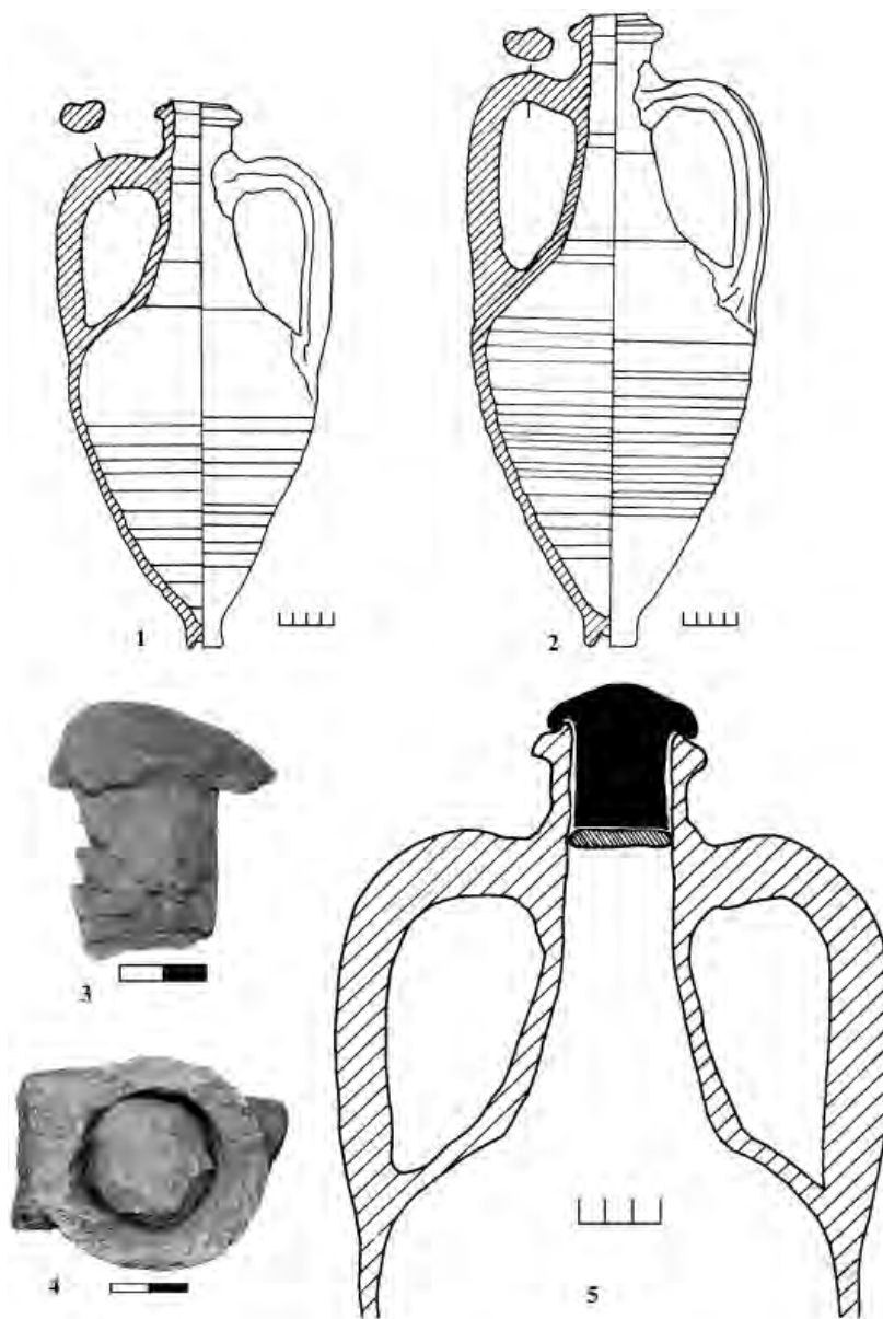
Рис. 5. 1 – амфора типа D из Танаиса (Т-99-ХІХ, пост. 4, пом. 7, № 244, 2535); 2 – амфора типа D из раскопок Хапровского городища (Х-97, р. II, п.І(4), амф. VIII № 178); 3 – глиняная пробка; 4 – горло амфоры со стопором; 5 – амфора D с пробкой и стопором (реконструкция).
