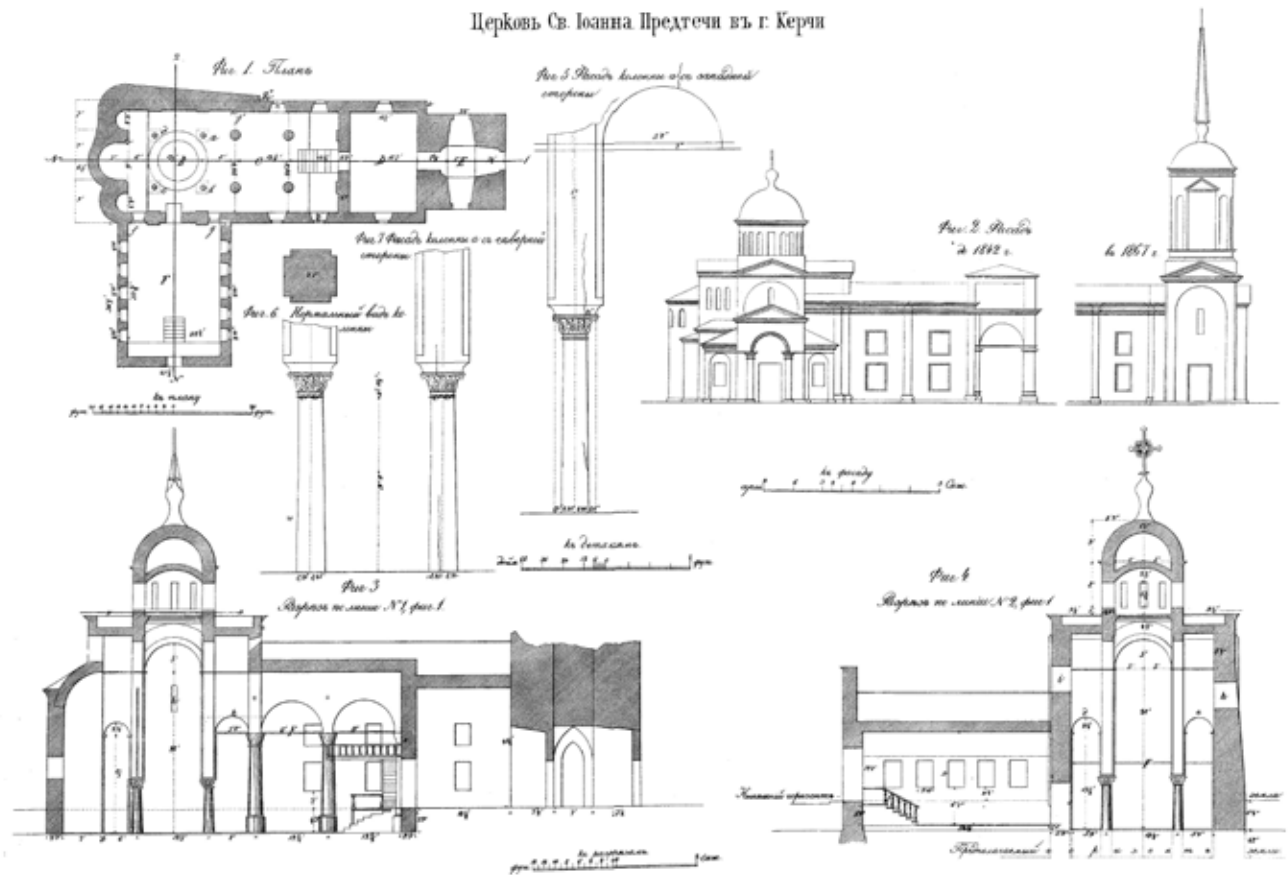
Рис. 3. Церковь Иоанна Предтечи. План, фасады, разрезы и архитектурные детали (по Рыздзевский, 1868).
