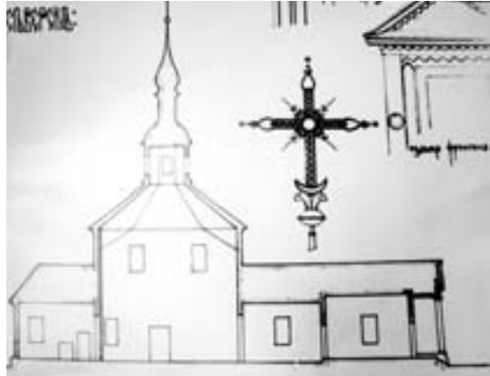
План церква св. Варвари з Новгород-Сіверського
