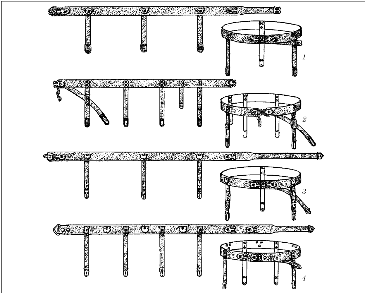
Рис. 6. Реконструкція поясних наборів з Т-подібними бляшками А.І. Куйбишева та В.В. Дорофеева: 1 — Роздольне, п. 5 к. 12; 2 — Василівка, п. 2 к. 2; 3 — Сивашівка, п. 2 к. 3; 4 — Чорноморське, п. 11 к. 1 (за: [Хардаев, 2015])
