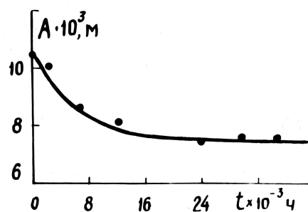
Рисунок 3 – Изменение амплитуды колебаний конвейера КВ2Т при длительной эксплуатации
