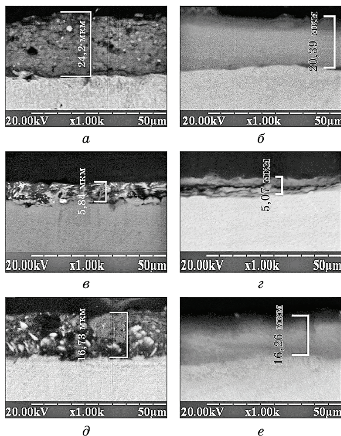
Рис. 4. РЕМ-зображення поперечних перерізів зразків сплаву ВТ6 після УЗУО з порошками \text{Al}_2\text{O}_3 (а, б), \text{Cr}_2\text{O}_3 (в, г) та їх суміші (д, е).
