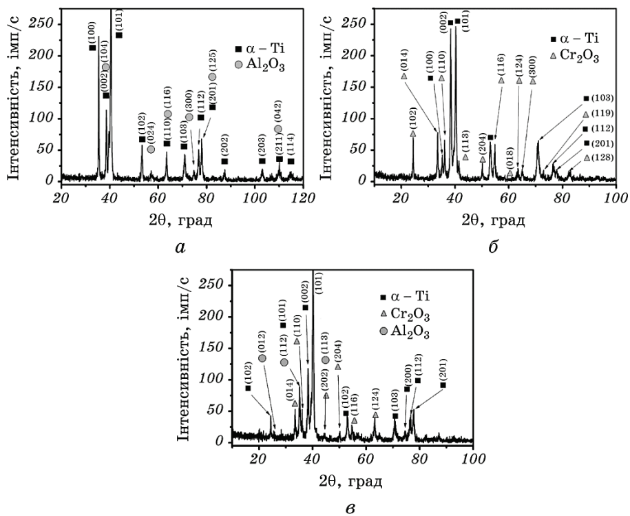
Рис. 3. Рентгенівські дифрактограми ступу ВТ6 після УЗУО з додаванням у зону деформації порошоків \text{Al}_2\text{O}_3 (а), \text{Cr}_2\text{O}_3 (б) та їх суміші (в).
