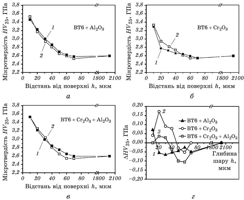
Рис. 7. Профілі мікротвердості (а, б, в) та їх зміни (г) у поперечному перерізі зразків ступу ВТ6 після УЗУО з порошками Al_2O_3 (а), Cr_2O_3 (б) та їх суміші (в) до (1) і після (2) високотемпературної витримки.
