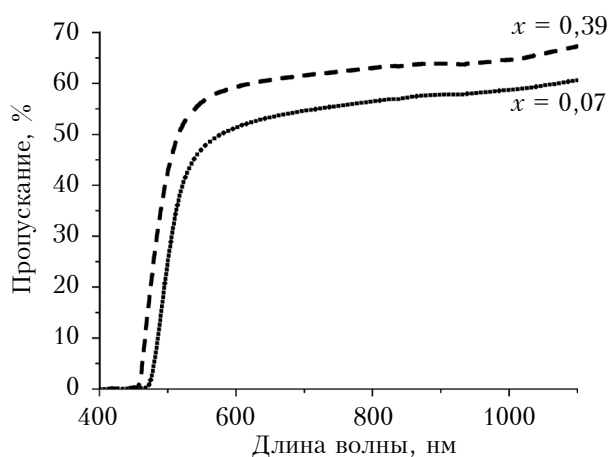
Рис. 1. Спектры оптического пропускания двух исследуемых образцов ZnS_xSe_{1-x} различного состава
