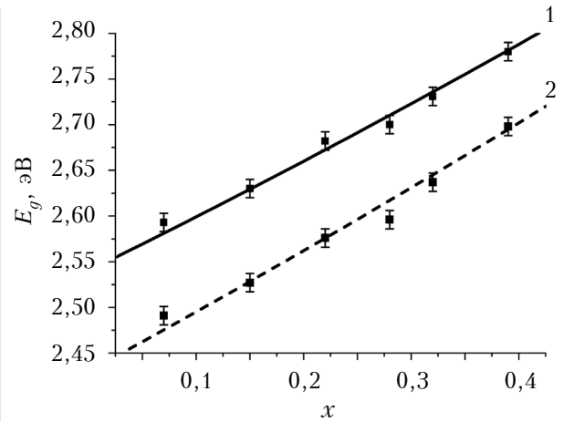
Рис. 3. Зависимость ширины запрещенной зоны от концентрации серы для прямых (1) и не прямых (2) переходов смешанных кристаллов ZnS_xSe_{1-x} (точки – экспериментальные результаты, полученные для шести исследуемых образцов; линии – зависимости, рассчитанные по уравнению (4))
