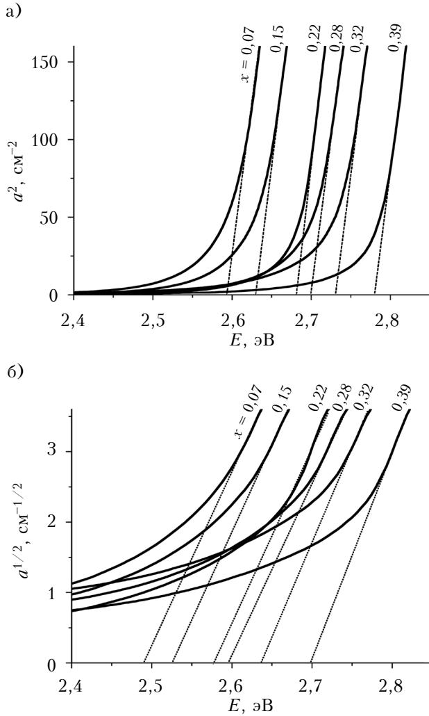
Рис. 2. Зависимость квадрата (а) и корня квадратного (б) коэффициента поглощения от энергии фотонов шести исследуемых образцов ZnS_xSe_{1-x} различного состава
