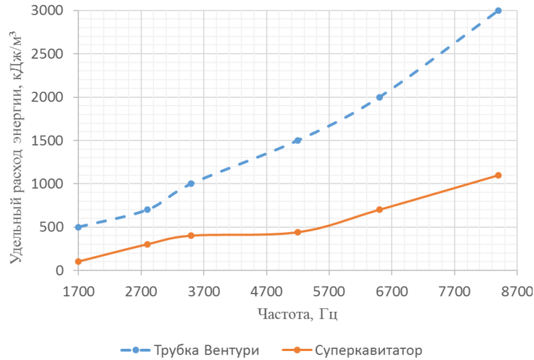
Рис. 4. Удельный расход энергии на кавитационном генераторе
