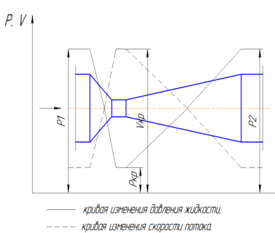
Рис. 1. Схема работы трубки Вентури
