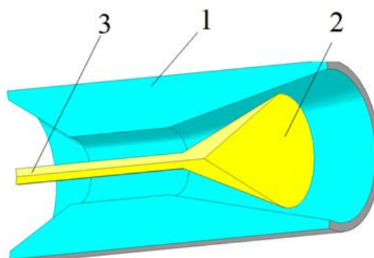
Рис. 3. Суперкавитационный генератор: 1 - ниппель специального сечения; 2 – конус обтекания; 3 – шток
