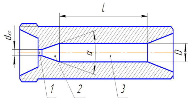
Рис. 2. Генератор импульсов давления (ГИД): 1 – критическое сечение генератора с минимальным диаметром; 2 – диффузор; 3 – последидиффузорный проточный канал
