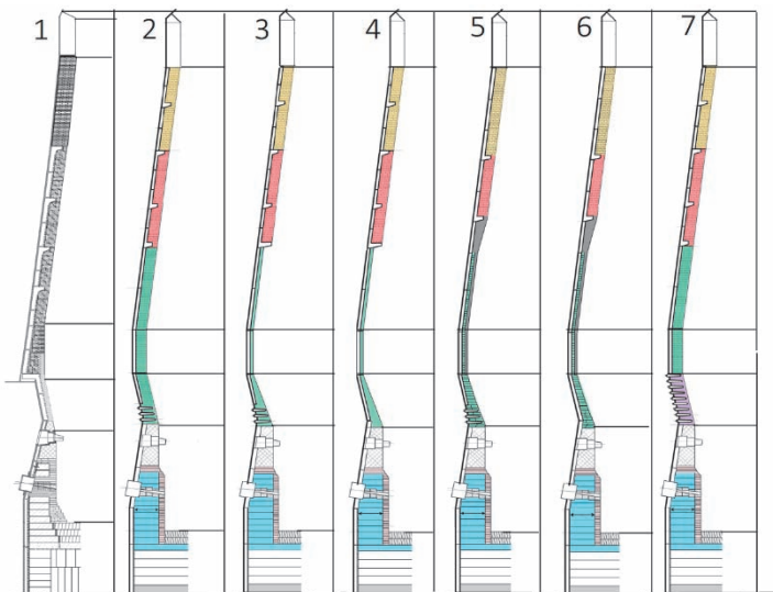
Рисунок 6 – Эскиз старого (1) и проектные варианты (2-7) конструкции профиля доменной печи полезным объемом порядка 2000 м 3 для работы с ПУТ
