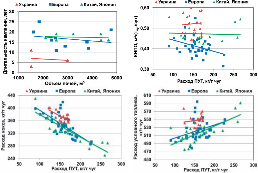
Рисунок 1 – Сопоставление с зарубежной практикой длительности кампании и лучших показателей работы с ПУТ доменных печей ПАО «Запорожсталь», ЧАО «ММК им. Ильича» и ПАО «АМК»
