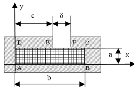
Рис. 2. Плоскопараллельная модель зоны обмоточного окна
