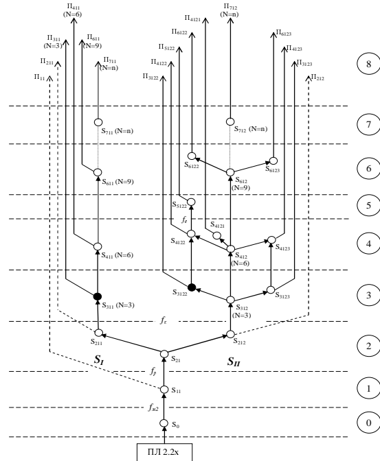
Рис. 1. Графическое представление дивергентной генетической модели (задача синтеза популяционной структуры плоских тяговых асинхронных двигателей (Вид ПЛ 2.2x) с групповой симметризацией фазных токов)
