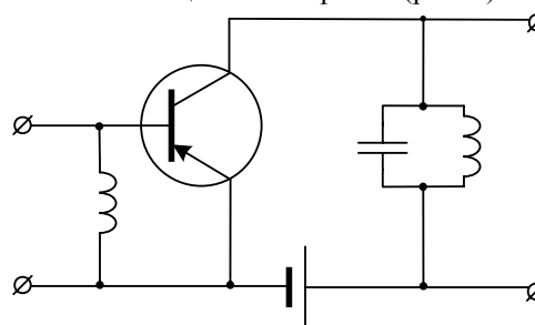
Рис. 6. Упрощенная схема усилителя мощности на полупроводниковом триоде
