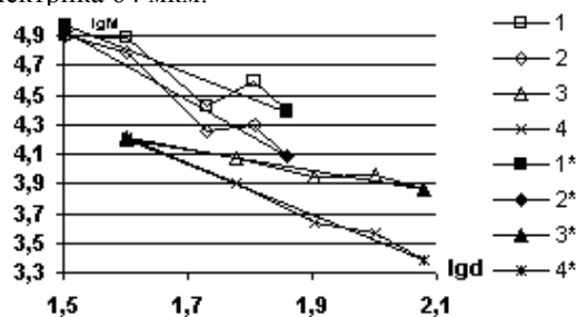
Рис. 1. Экспериментальные зависимости (\lg M)_{ср} от толщины диэлектрика \lg d для герметичных (1) и негерметичных (3) секций и приведенные к постоянному числу слоев диэлектрика (2) и (4) при N=4
