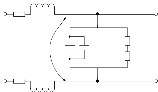
Рис.2. Схема замещения увлажненного кабеля
