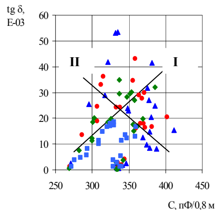
Рис.7. C - \text{tg}\delta зависимости образца кабеля в процессе увлажнения для разных частот
