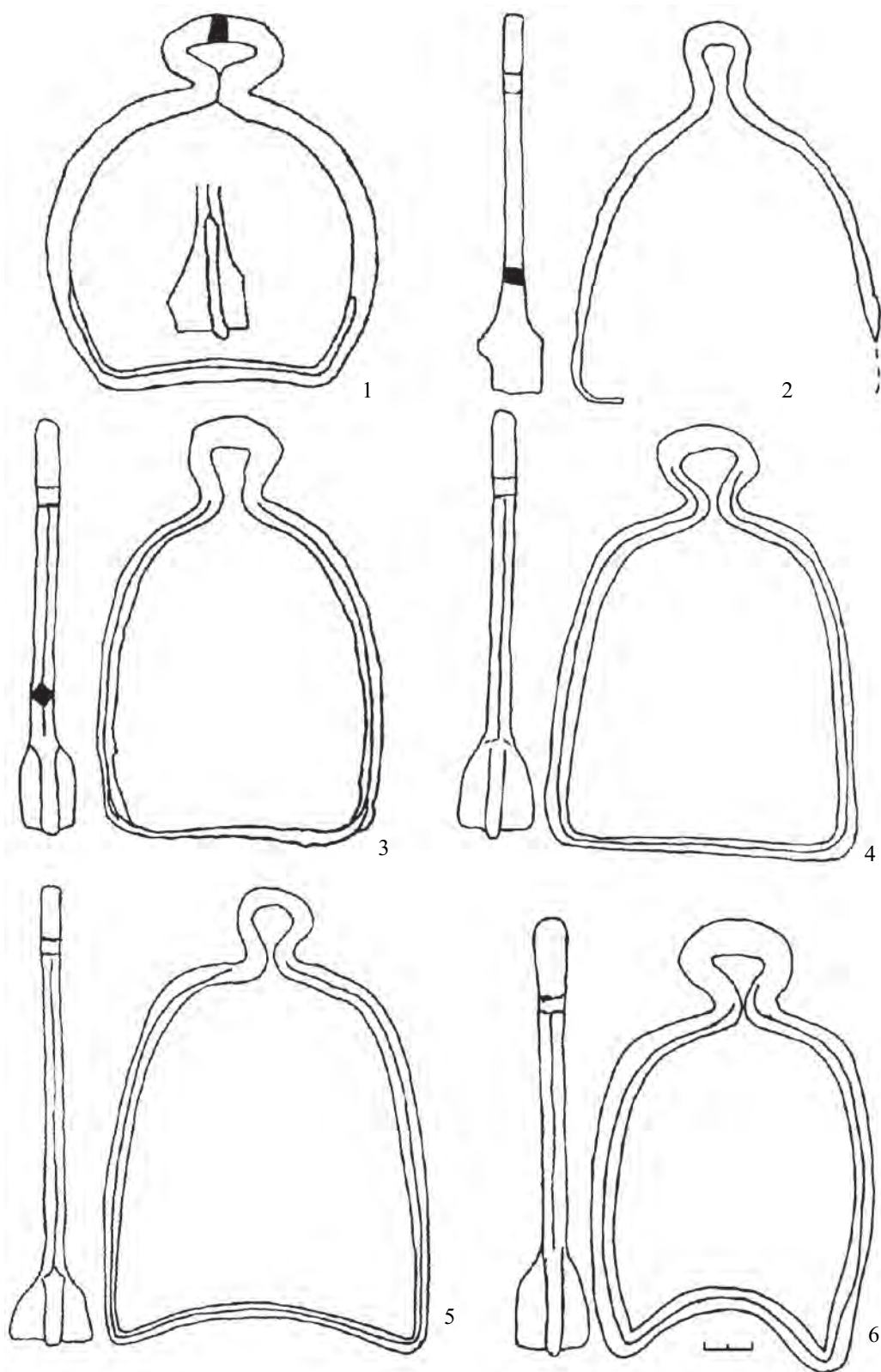
Рис. 41. Стремена (окончание): 1 – Шелехметь II, к.11, п.4; 2 – Шелехметь II, к.1; 3-5 – Брусяны II (3 – к.12, п.2; 4 – одиночный курган, п.2; 5 – к.23, п.6); 6 – Новинки II, к.14, п.4.
