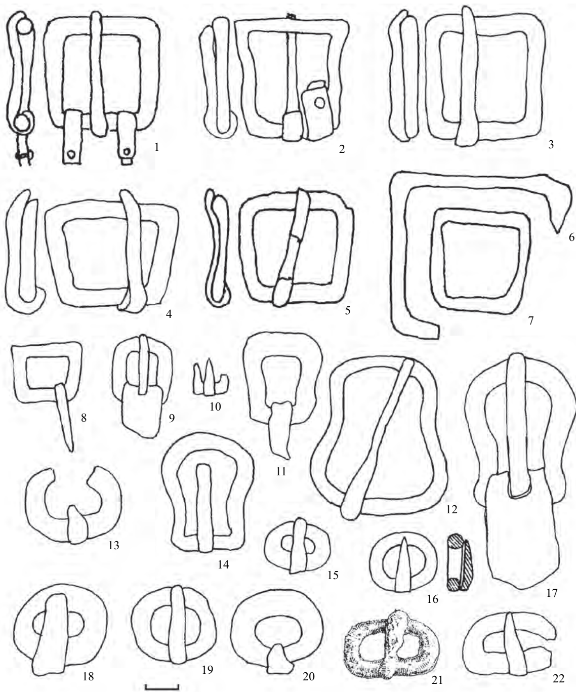
Рис. 47. Железные пряжки: 1, 3 – Заплавка; 2, 4, 5, 8, 12 – Вознесенка; 6, 7 – Глодосы; 9, 15, 19 – Наташино, к.17; 10 – Старонизхестеблиевская; 11, 20 – Калининская (11 – к.30, п.3; 20 – к.4, п.10); 13 – Малая Терновка, к.24, п.3; 14, 17 – Уч-Тепе; 16 – “Царский курган”; 18 – Портовое; 21 – Аджиголь; 22 – Васильевка, к.2, п.1.
