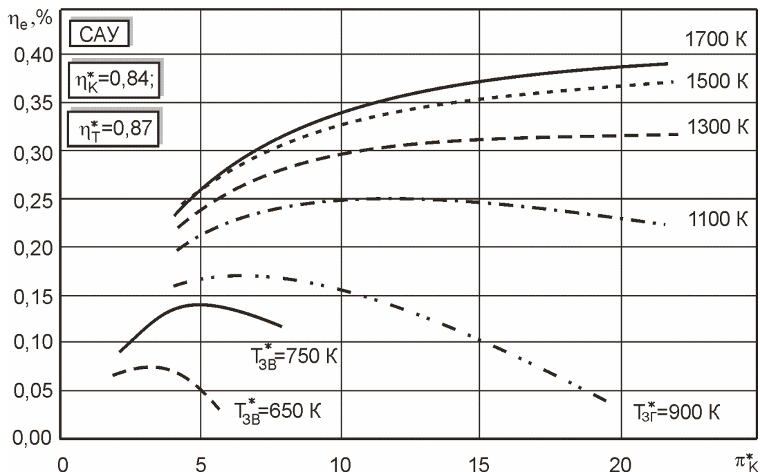
Рис. 3. Влияние параметров цикла ГТТ на его энергетический КПД.
