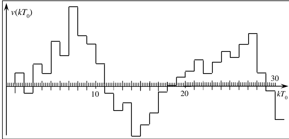
Рис. 1. График марковского процесса v[(k + 1)T_0] = gv(kT_0) + \zeta(kT_0) при g = 0,85
