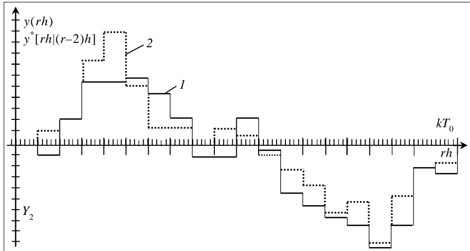
Рис. 2. Графики моделирования выходной переменной (1) и ее прогнозируемого значения (2) на основе функции прогнозирования без приращения переменных
