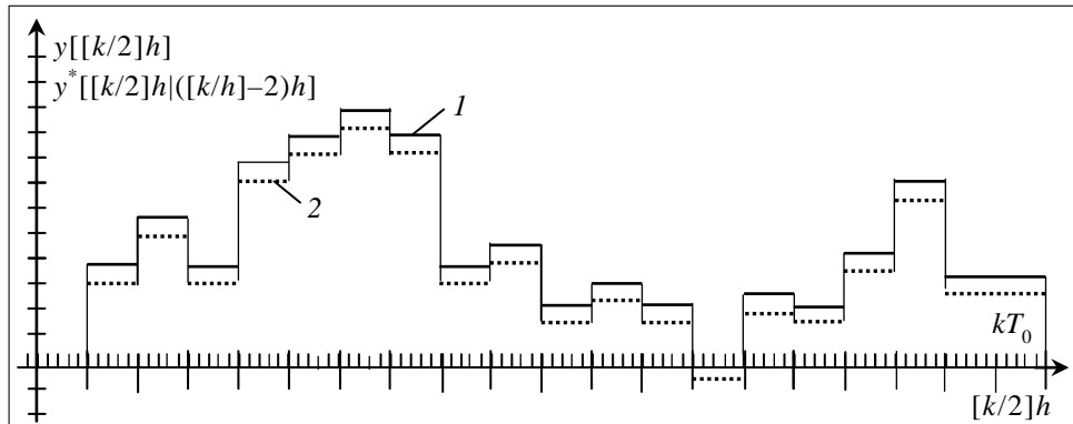
Рис. 3. Графики моделирования выходной переменной (1) y[[k/2]h] и ее прогнозируемого значения (2) на основе функции прогнозирования в приращениях переменных
