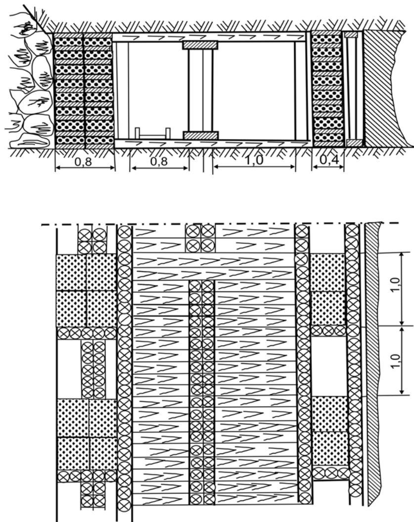
Рис. 2. Паспорт крепления вентиляционной печи для условий пласта m_3 «Голстый» на ш. «Северная»
