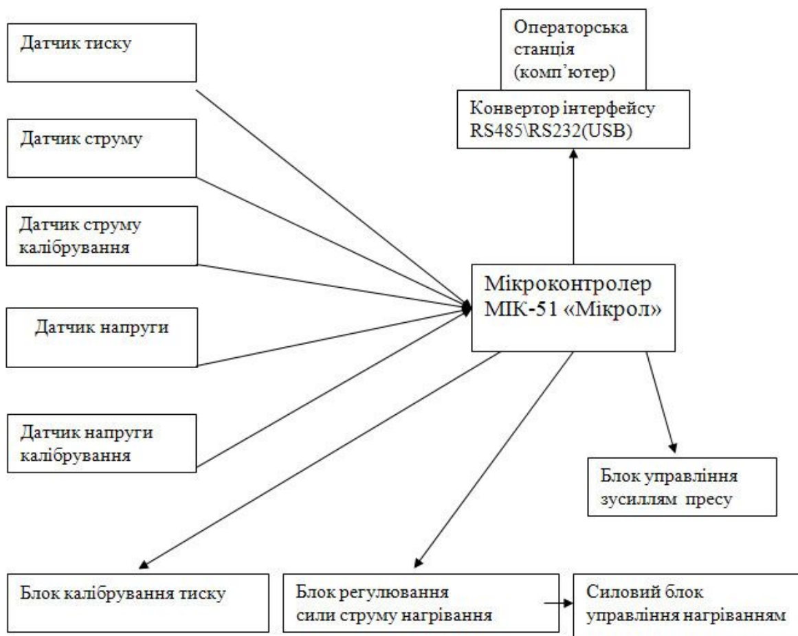
Рис. 1. Структура автоматизованої системи управління процесом спікання
