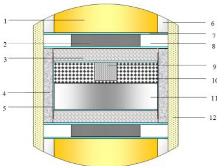
Рис. 3. Схема спорядження КВТ для вимірювання кінетики просочування алмазного мікропорошку розплавом Co-W-C_{алм} з підкладки BK15: 1 – шайба з пірофіліту; 2 – графітовий диск; 3 – диск з VN_{гр.} ; 4 – графітовий нагрівач; 5 – молибденовий екран; 6 – графітовий струмопідвід; 7 – фольга з термографеніту; 8 – кільце з пірофіліту; 9 – диск з молибдену; 10 – алмазний мікропорошок АСМ 40/28; 11 – підкладка з BK15; 12 – фрагмент контейнеру з літографського каменя
