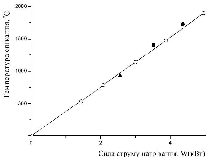
Рис. 5. Залежність температури спікання від сили струму нагріву (при тиску 8,0 ГПа: ▲ – плавлення кремнію; ■ – плавлення міді; ● – плавлення нікелю)
