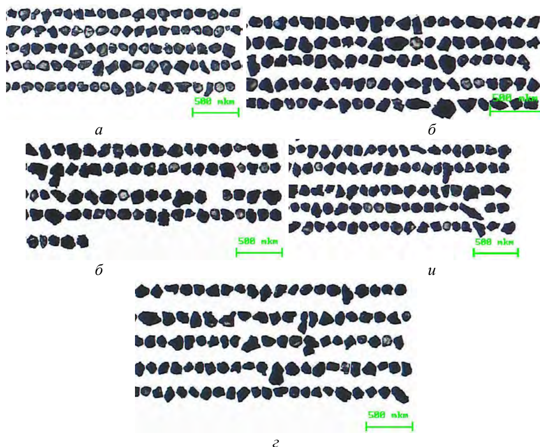
Рис. 1. DiaInspect-фотографии зерен шлифпорошков AC20 100/80 исходного (а), металлизированных Ni (б) и Cu (в) и композиционными покрытиями Ni-Al (г) и Cu-Al (д)
