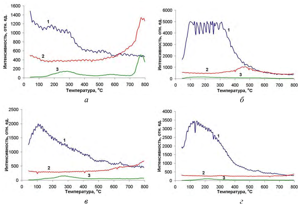
Рис. 2. Термодесорбционные кривые шлифпорошков AC20 100/80, металлизированных Ni (а), Cu (в) и композиционными покрытиями Ni–Al (б), Cu–Al (г): 1 – паров воды на поверхности зерен алмазов; 2 – монооксида углерода CO; 3 – диоксида углерода CO 2
