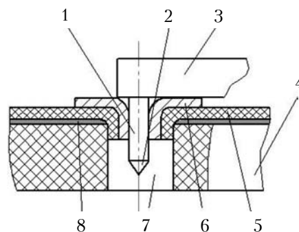
Рис. 1. Контактное соединение
