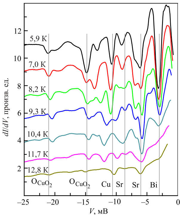
Рис. 6. (Онлайн в цвете) Фрагмент спектра динамической проводимости SIS контакта на микротрещине в недодопированном образце Bi-2201(La) с T_c \approx 21 К в интервале температур 5,9–12,8 К. Положение особенностей, вызванных взаимодействием переменного джозефсоновского тока с оптическими фононными модами, отмечено вертикальными линиями. Взято из [113].
