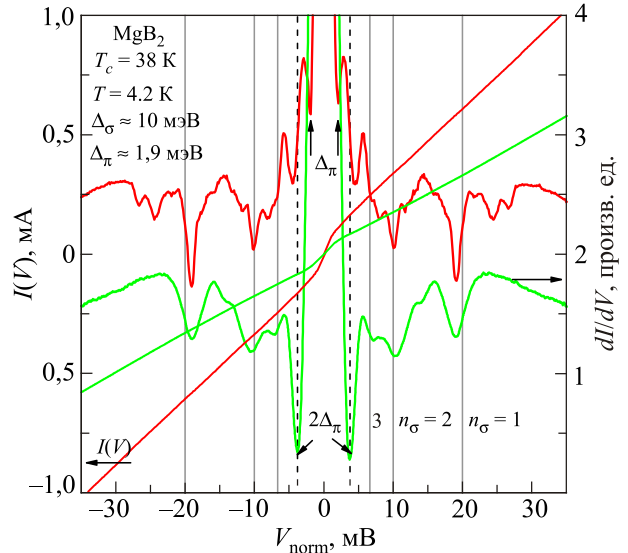
Рис. 9. (Онлайн в цвете) Нормированные по смещению на один контакт ВАХ (левая вертикальная ось) и dI(V)/dV -спектры (правая ось) андреевских SnSn...S структур (верхний спектр — m = 5 контактов, нижний спектр — m = 2 ), полученных на образцах MgB_2 из одной закладки с T_c \approx 40 К. T = 4,2 К. Минимумы СГС от большой щели \Delta_\sigma \approx 10 мэВ отмечены серыми вертикальными линиями и значками n_\sigma = 1, 2, 3 ; СГС от малой щели \Delta_\pi \approx 1,9 мэВ — пунктиром и стрелками.
