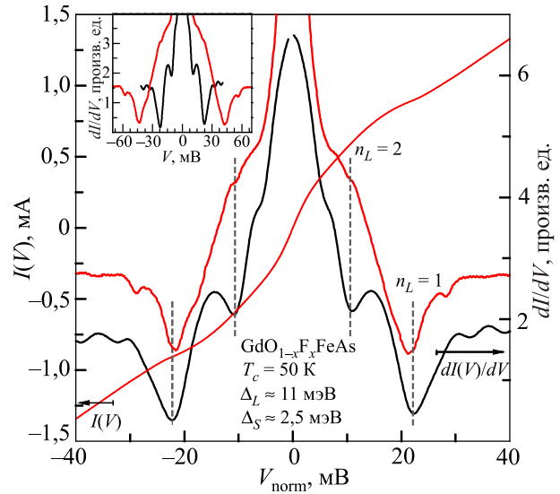
Рис. 14. (Онлайн в цвете) Динамическая проводимость одиночного SnS контакта (черная кривая), а также нормированные (красные кривые) ВАХ (левая вертикальная ось) и dI(V)/dV -спектр (правая вертикальная ось) двухконтактной стопки, полученные в оптимально допированных образцах \text{GdO}_{1-x}\text{F}_x\text{FeAs} с T_c \approx 50 К. T = 4,2 К. Положения СГС для большой щели \Delta_L \approx 11 мэВ показаны штриховыми линиями и значками n_L = 1, 2 . На вставке приведены данные спектры до нормировки.
