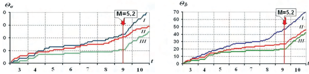
Рис. 4. Кумулятивна сейсмічність з 3-ї по 10-ту годину 27.09.2004 р., розрахована за результатами дисперсійного аналізу (а) та АФР (в) для САЗ: I – Вранча; II – Закарпаття; III – Крим.
