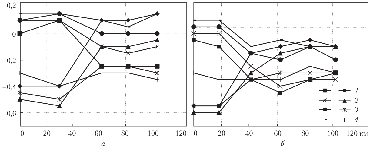
Рис. 2. Графики поведения компонент вещественных типперов ReW_{СЮ,ВЗ} для периодов: 1 – 10 с; 2 – 300 с; 3 – 800 с; 4 – 2200 с по профилям Кагарлык–Черкассы (а), Головуров–Гребенка (б)
