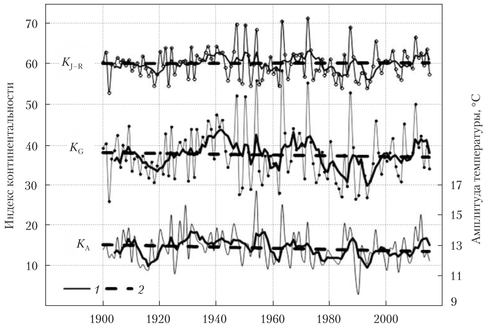
Рис. 2. Вековой ход индексов континентальности ( K_G и K_{J-R} ) и амплитуды сезонного хода температуры ( A ) на территории Украины за период 1900–2015 гг. (1 – скользящее усреднение, 2 – линейный тренд)
