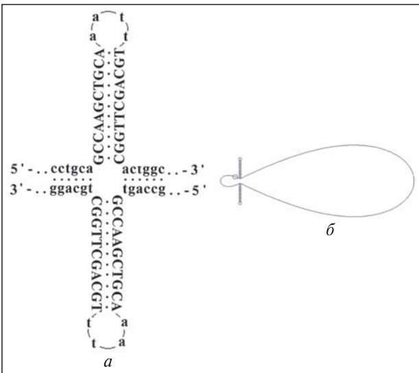
Рис. 3. Хрестоподібна структура суперспіральної плазміді рUC8, отримана за допомогою пакета прикладних програм GeneVee: a – фрагмент послідовності ДНК рUC8 (позиції 273–298), який набуває хрестоподібної структури; б – хрест, який утворюють інвертовані повтори ДНК плазміді рUC8
