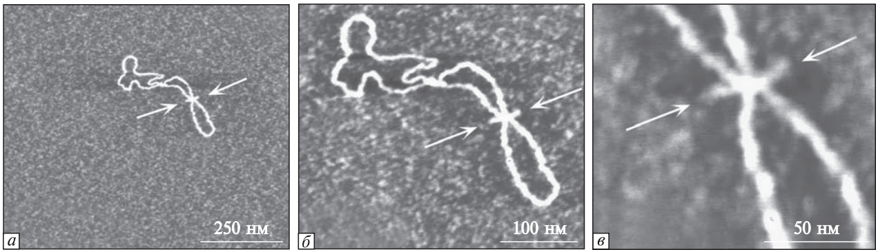
Рис. 2. АСМ-зображення суперспіральної плазміді рUC8 (довжина становить 2665 п.н.) у повітрі. Розмір кадру: a – 858 × 858 нм; б – 372 × 372 нм; в – 134 × 134 нм. Стрілками показано дві шпильки, що утворюють хрестоподібну структуру
