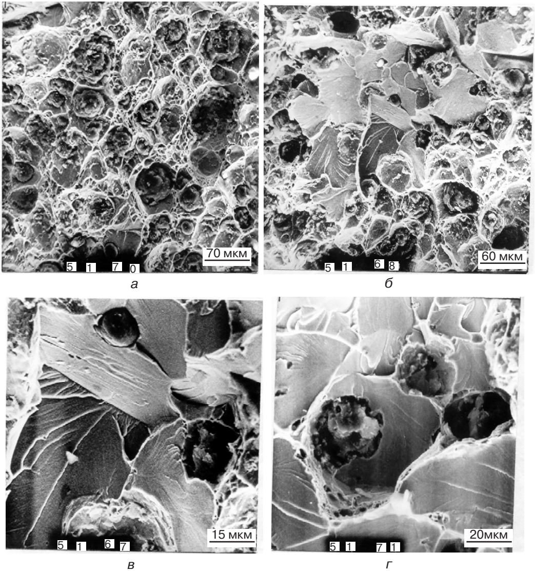
Рис. 2. Микрофотографии изломов (фрактограммы) образцов чугуна плавки 3 при температуре 0 °С: а – вязкий излом; б – вязко-хрупкий; в, г – в основном хрупкий, РЭМ
