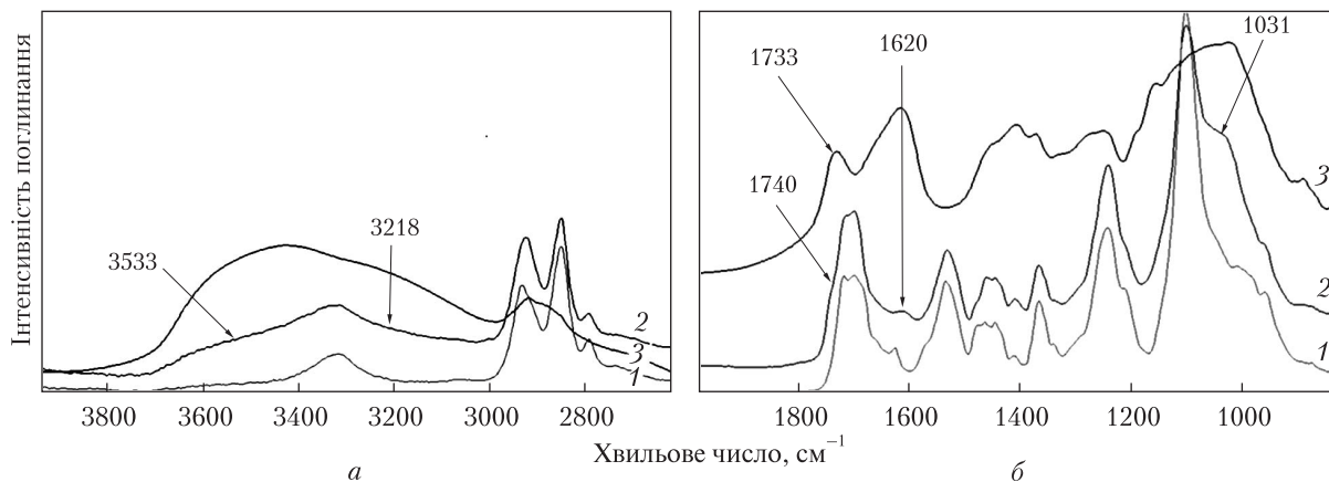
Рис. 2. ІЧ спектри ІПУ (1), ІПУ/РО/Кс (2), Кс (3)
