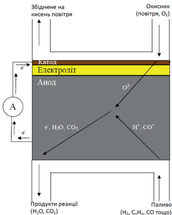
Схематичне зображення роботи керамічної паливної комірки
