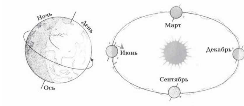
Рис. 7. Обращение Земли вокруг Солнца. Эксцентриситет орбиты e=0,0167 , c=2,5 млн км, афелий в июле составляет 152,1 млн км, V_a=29,6 км/с, перигелий в январе — c=147,1 млн км, V_p=30,1 км/с. Ось вращения эллиптической земной орбиты для весны и осени — 149,6 млн км, V=29,85 км/с.
