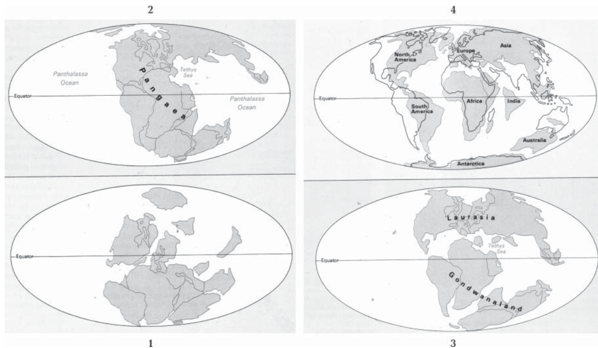
Рис. 10. Эволюция дрейфа материковых тектонических плит: 1 — 360 млн лет назад (карбон), 2 — 180 млн лет назад (юра), 3 — 120 млн лет назад (мел), 4 — 60 млн лет назад (палеоцен и современность); [World..., 2000].
