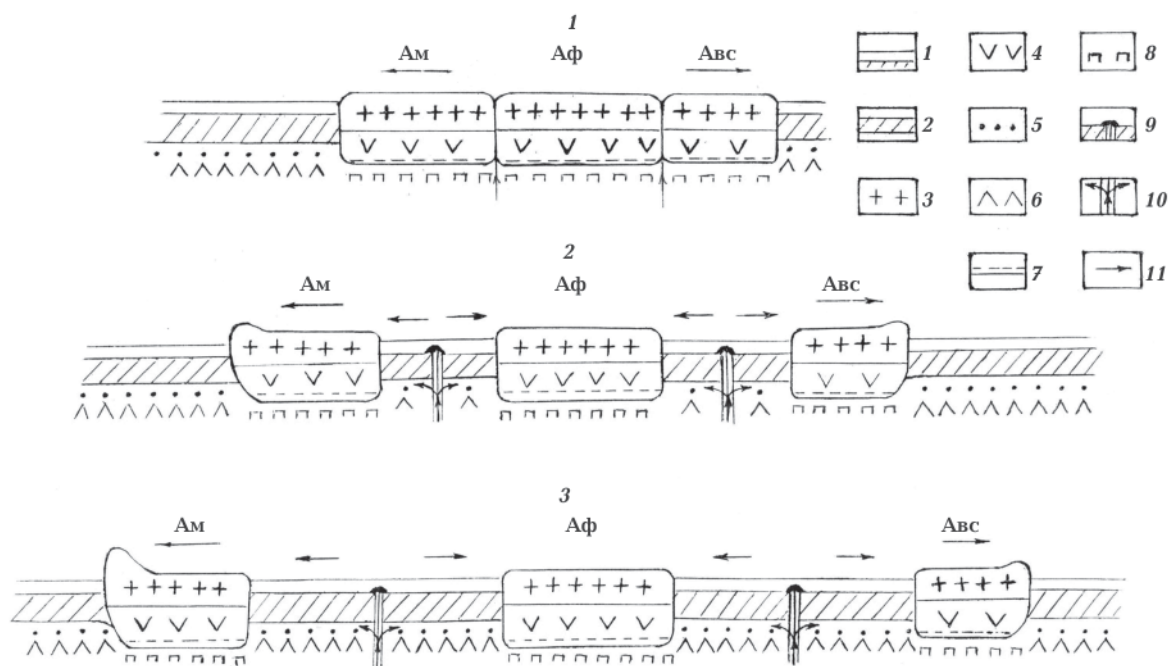
Рис. 8. Принципиальная схема дрейфа литосферных плит при раскрытии Атлантического и Индийского океанов: I — мезозой — юра, мел (возраст 135—150 млн лет); II — начало кайнозоя (65 млн лет), в — современность; 1 — океан над океанической плитой; 2 — габбро-базальтовая океаническая плита; III — гранитная часть материковой плиты; 4 — габбровая часть материковой коры; 5 — магматическая базальтоидная подошва океанической плиты; 6 — океаническая ультрабазитовая мантия; 7 — материковая перидотитовая мантия; 8 — срединно-океанический хребет; 9 — раздвижение океанических плит по срединно-океаническому рифту; 10 — тальк-серпентинитовая подошва материковых плит; 11 — направление (вектор) движения плит. Материковые плиты: Ам — Америка, Аф — Африка, Авс — Австралия. Между Африкой и Америкой — Атлантический океан, а между Африкой и Австралией — Индийский.
