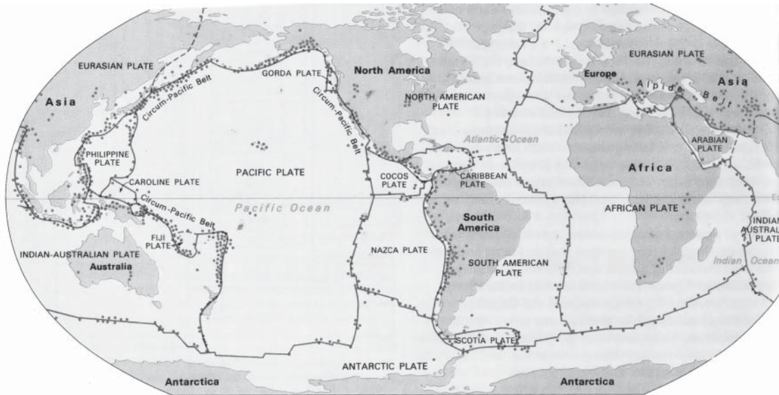
Рис. 1. Крупные землетрясения приурочены к границам дрейфующих тектонических плит.
