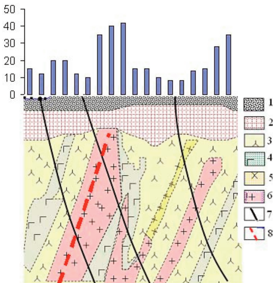
Рис. 3. Геологический разрез Полоховского участка. 1 – песок среднезернистый, 2 – суглинки, 3 – гнейсы, 4 – граниты, 5 – граниты аплит-пегматитовые, пегматиты, 6 – граниты аплит-пегматитовые с богатым оруденением, 7 – скважины, 8 – тектонические нарушения
