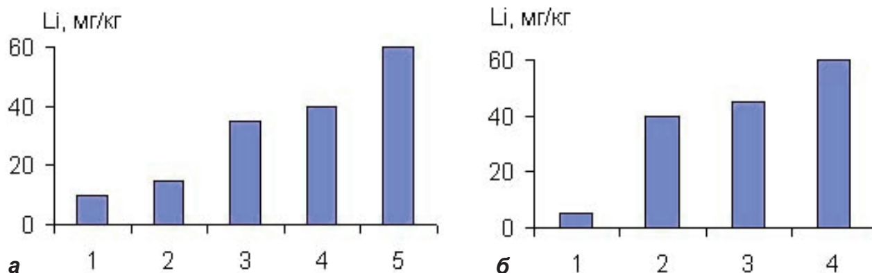
Рис. 1. Содержание лития в породах Украинского щита: а – кристаллических (1 – ультраосновные, 2 – основные, 3 – средние, 4 – кислые, 5 – щелочные); б – осадочных (1 – известняки, 2 – песчаники, 3 – алевриты, 4 – аргиллиты)
