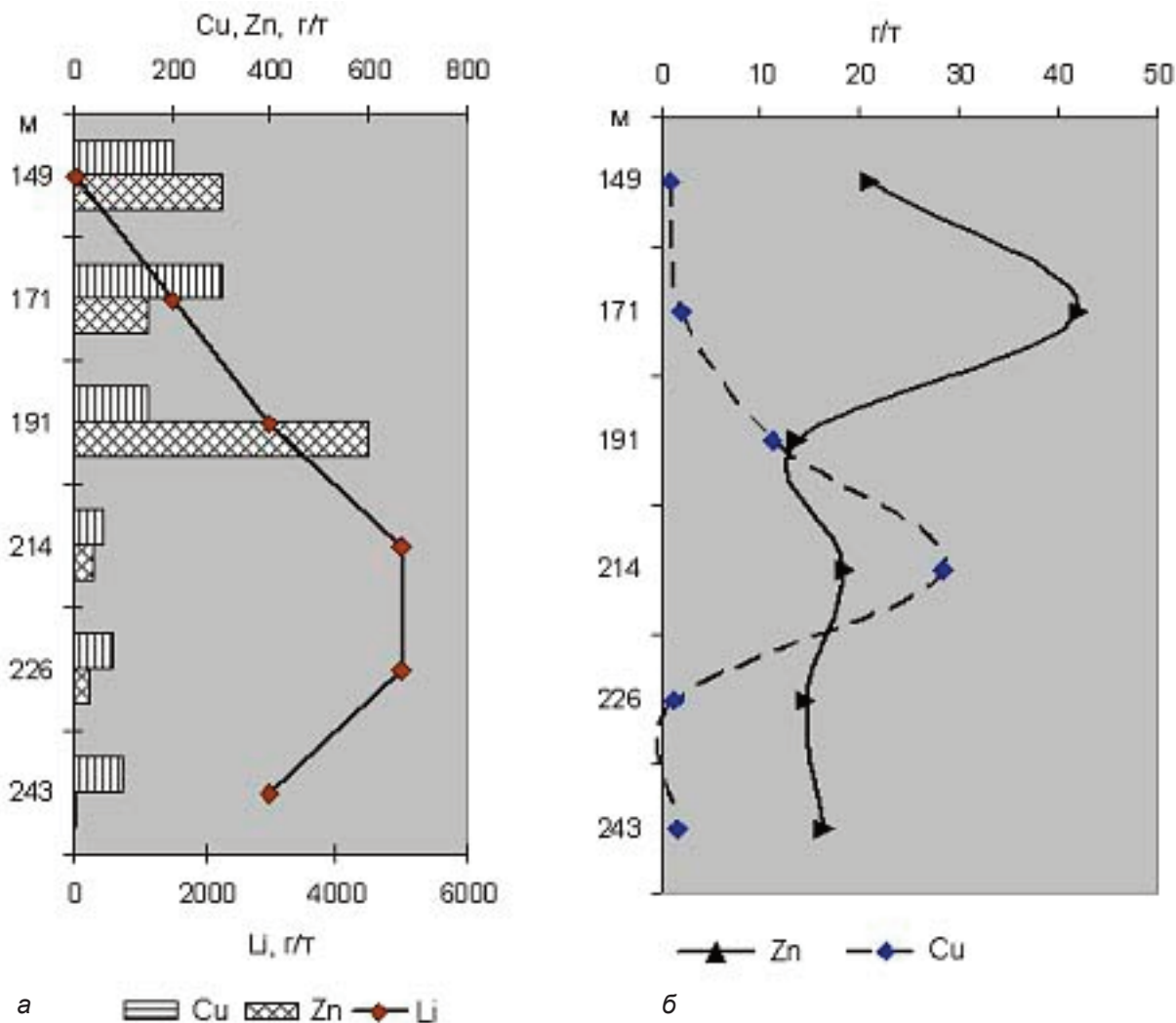
Рис. 2. Содержание валовое (а) и степень подвижности (б) химических элементов в вертикальном разрезе Полоховского месторождения
